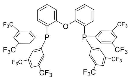
3,5- \text{CF}_3\text{DPEPhos}
